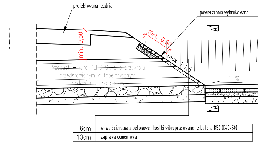
SZCZEGÓL 7.2 WYBRUKOWANA POWIERZCHNIA SKARPY WOKÓŁ WLOTU I WYLOTU PRZEPUSTÓW POD DROGAMI PRZEKRÓJ WLOTU/WYLOTU
